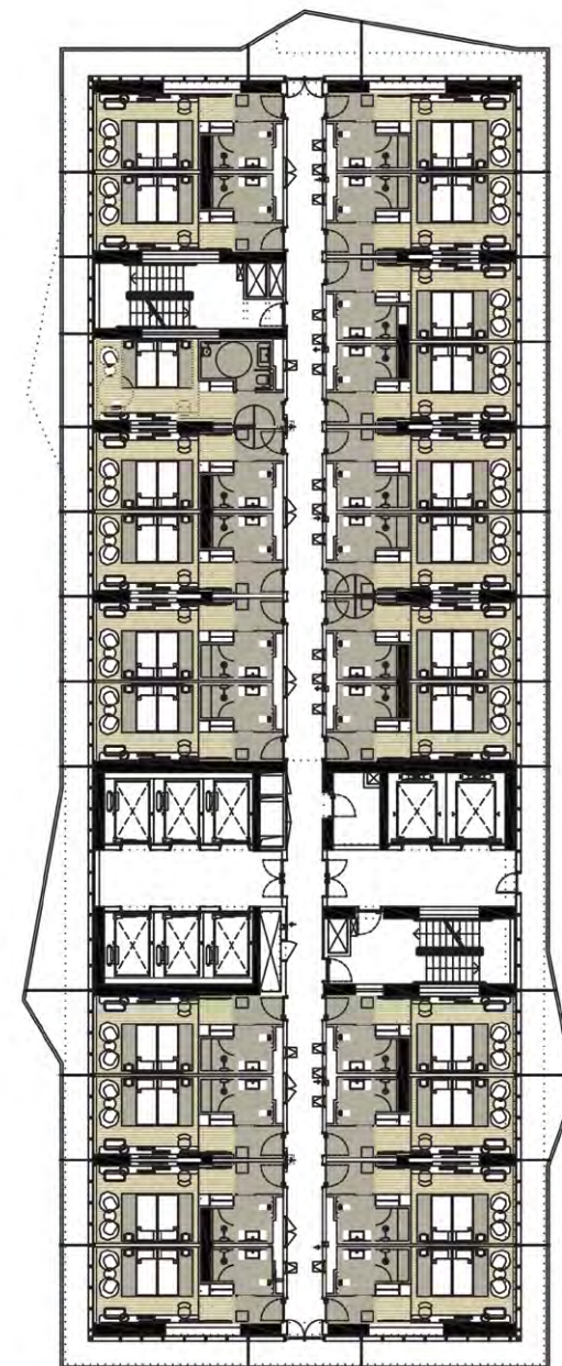
План этажа
